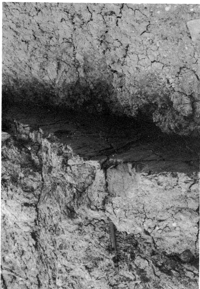
Fig. 5. La capa de margas se desliza sobresaliendo unos 35 cm sobre una de lutita (diciembre de 1991), en la margen derecha del arroyo Tlaxómotl.
