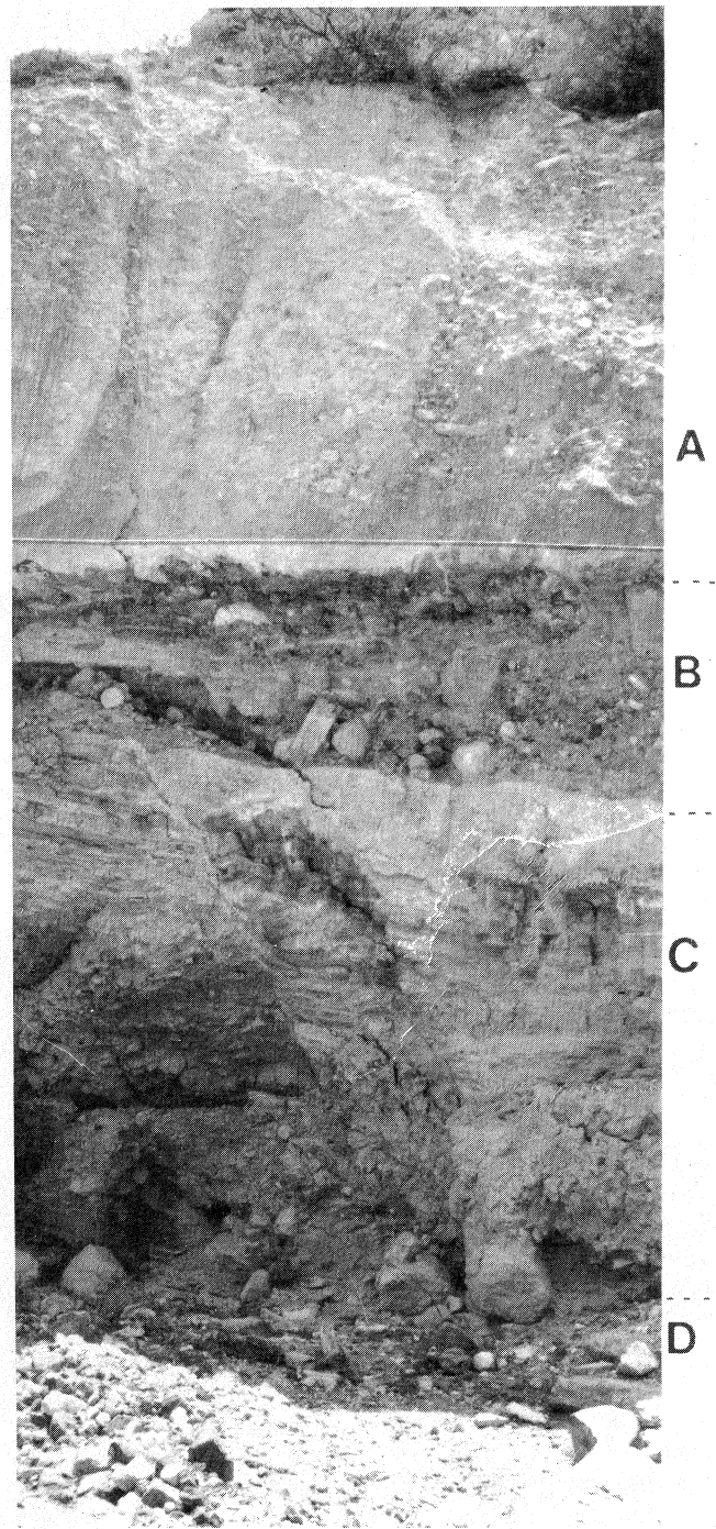
Fig. 3. Columna litológica que muestra la constitución del subsuelo de Mezquitlán. A, material detrítico depositado por corriente de lodo; B, cantos y bloques de cauce antiguo; C, estratos de margas y lutitas de la Formación Méndez; D, depósitos actuales de cauce.
