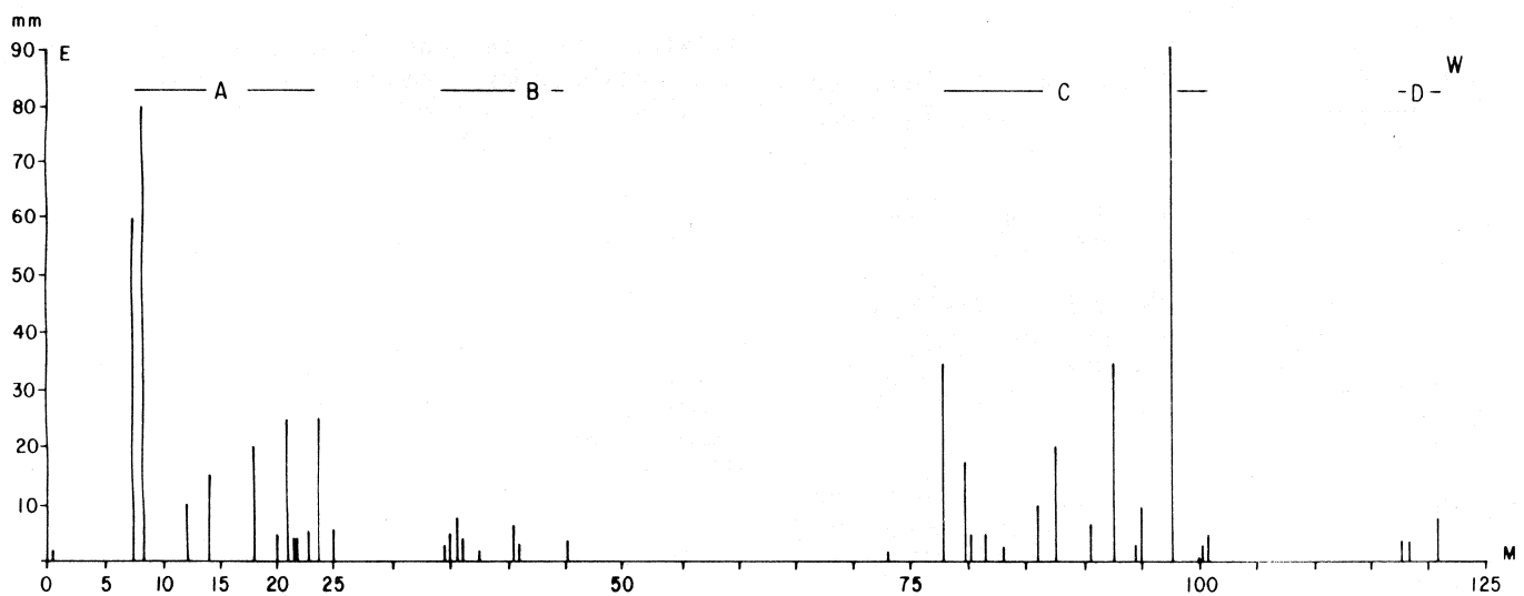
Fig. 14. Grietas en la calle Vasco de Quiroga. La escala vertical corresponde a los milímetros de abertura. A y C, expresan zonas de grieta maestra con clara expresión; B, con menor desarrollo, y D, inicio aparente. Mediciones hechas el 3 de octubre.
