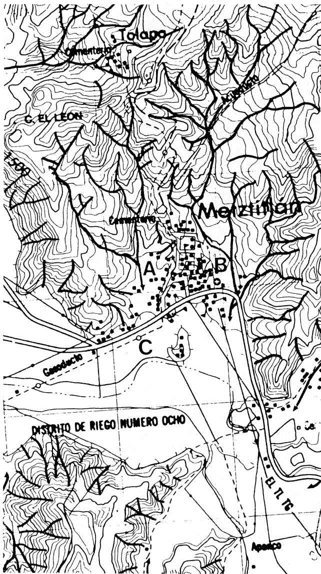
Fig. 2. La población de Mezquitlán (hoja F14061, 1:50,000) en una colina bordeada por dos arroyos (A y B - Tlaxómotl) que desembocan en la vega (C).
