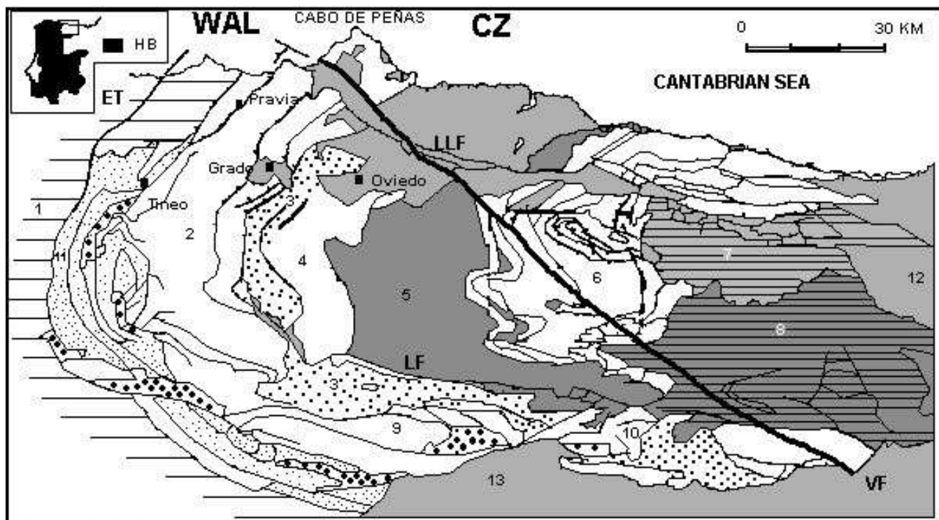
Fig. 4. Geological scheme of Cantabrian zone. [1: Zona Asturoccidental-Leonesa, 2: Unidad de Somiedo, 3: Unidad de La Sobía-Bodón, 4: Unidad del Aramo, 5: Cuenca Carbonífera Central, 6: Región del Ponga, 7: Picos de Europa, 8: Unidad del Pisuerga-Carrión, 9: Unidad de Correcilla, 10: Esla, 11: Cangas de Narcea, 12: Cuenca Vasco-Cantábrica, 13: Cuenca del Duero. CZ= Cantabrian Zone; ET= Espinar thrust; HB= Hercynian Belt in Western Iberia; LF= León fault; LLF= Llanera fault; VF= Ventaniella fault; WAL= Western Asturias-León Zone. Modified of Instituto Geológico y Minero de España, 1974].
