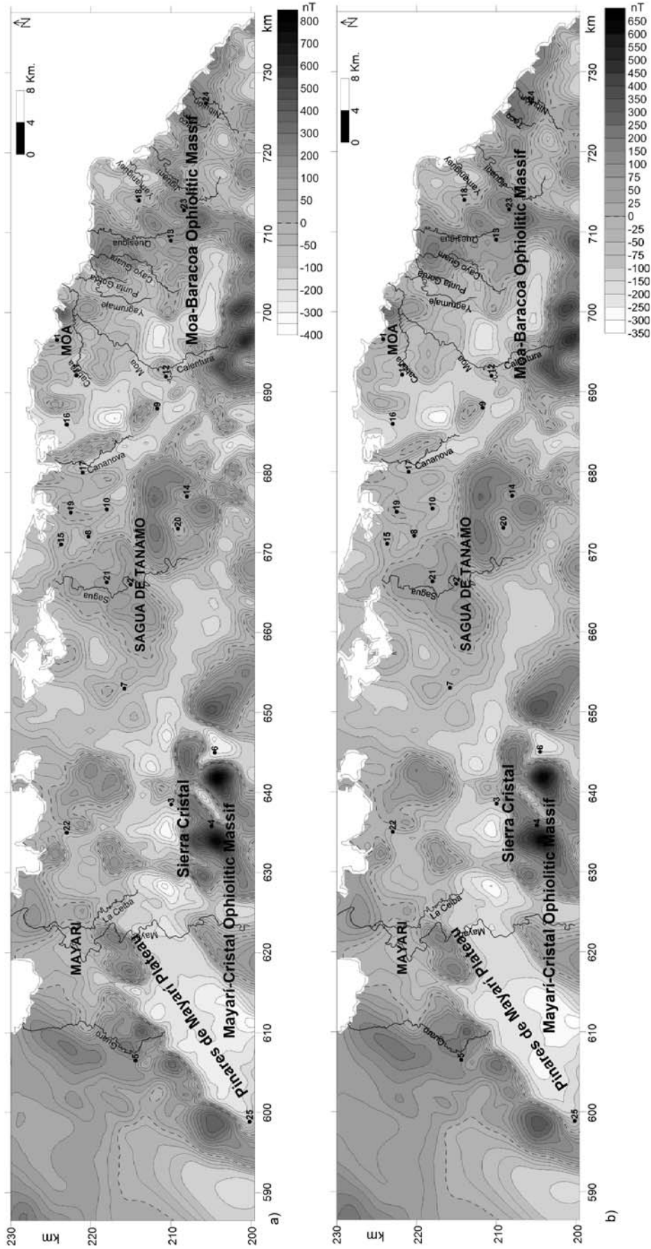
Fig. 10. Upward Continuation Map of the Mayarí-Sagua-Moa region. a, h=250 m; b, h=500 m; c, h=750 m; d, h=1500 m; e, h=1800 m; f, h=2200 m; g, h=4000 m. Towns: 1, Moa; 2, Sagua de Tanamo; 3, Sierra Cristal; 4, Cayo Verde; 5, Guamutas; 6, Moreiro; 7, La Güira; 8, Quemado de Aguacate; 9, Caïmanes; 10, Barbarú; 11, Centeno; 12, Calentura Abajo; 13, Quemado del Negro; 14, Hato Viejo; 15, Cayo Acosta Dos; 16, Yaguaneque; 17, Cananova; 18, Cayo Grande; 19, Melena Ocho; 20, Castro; 21, Paso de la Vacca; 22, Levisa; 23, La Penda; 24, La Vega de Taco; 25, Sierra de Nipe.
